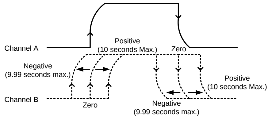
Fig. 延迟功能
