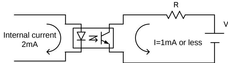
Fig. 光电耦合器 电流
