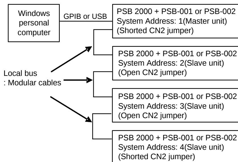
Fig. 本地总线连接
