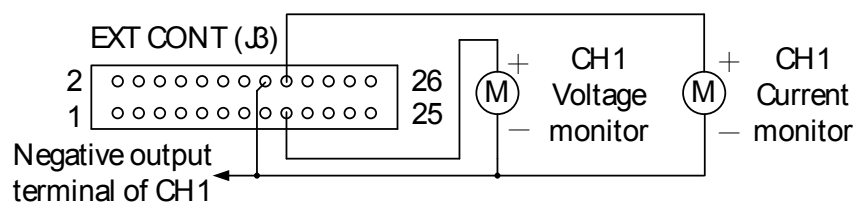
Fig. 监控输出引 脚
