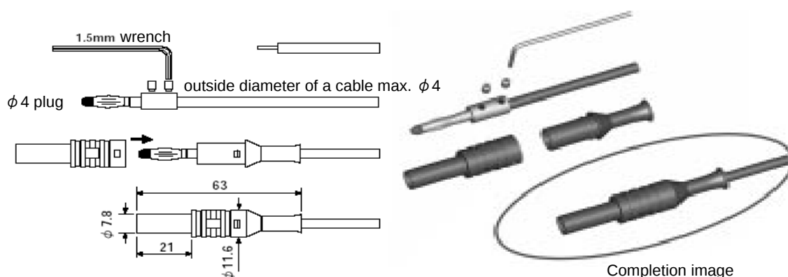
Fig. 前输出端插头的装配图
