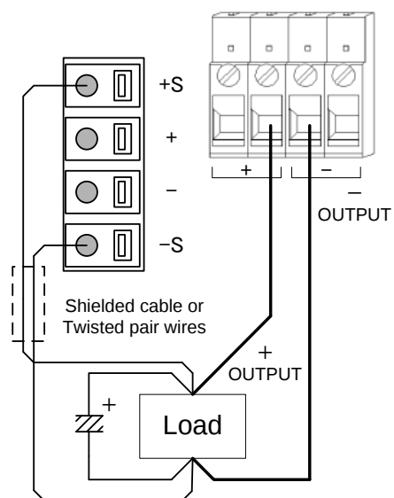
Fig. 远程传感连接 (PSB-H)
