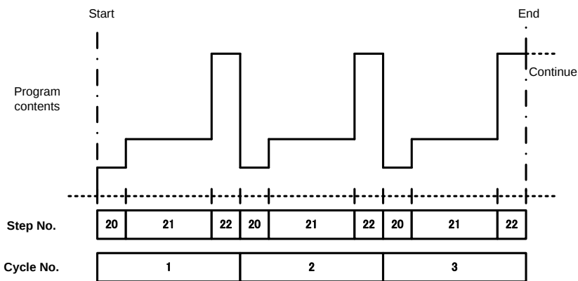
Fig. 重复 3 次 Step 20~22. 起始步 Step 20
