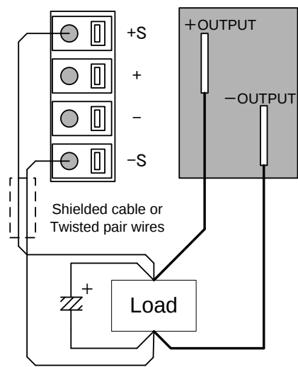
Fig. 远程传感连接 (PSB-L)
