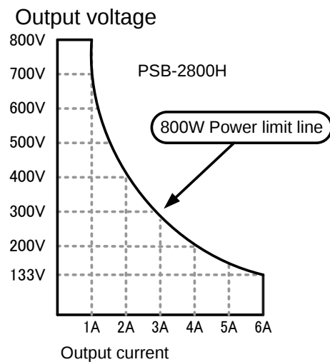
PSB-2800H 工作范围
