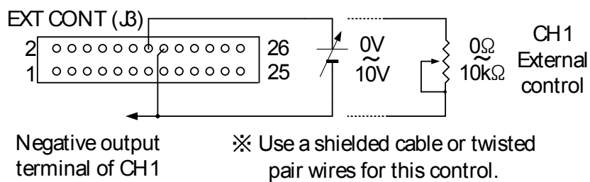
Fig. 外部电压/电阻控制端(CV)
