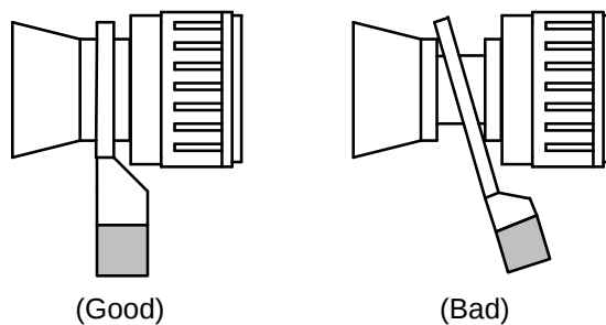
Fig. 连接前输出端
