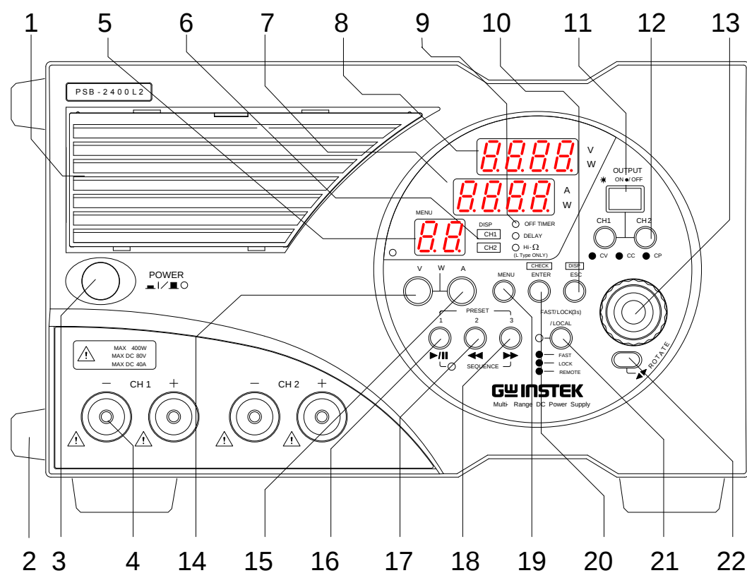
前面板(PSB-2400L2)
