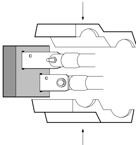
Fig. 合上后输出 端保护盖
