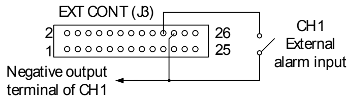
Fig. 外部报警输入引脚
