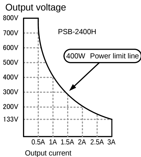
Fig. PSB- 2400H 工作范围
