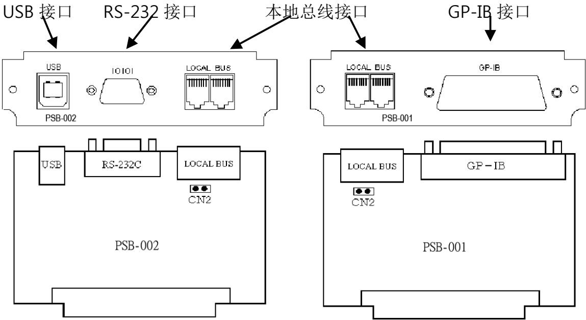
Fig. 接口示意图
