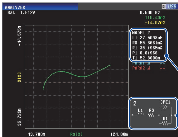
等效电路分析界面(锰干电池)
