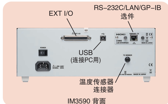
IM3590 背面
