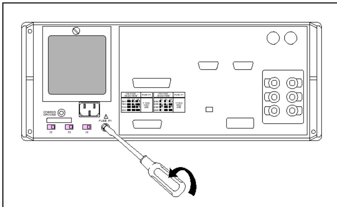
图7-1. 拆装保险丝
