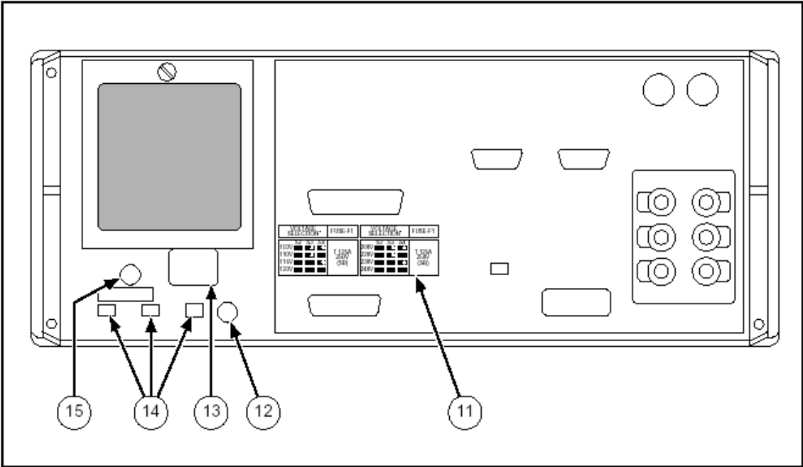
图3-2. 后面板功能（续）
