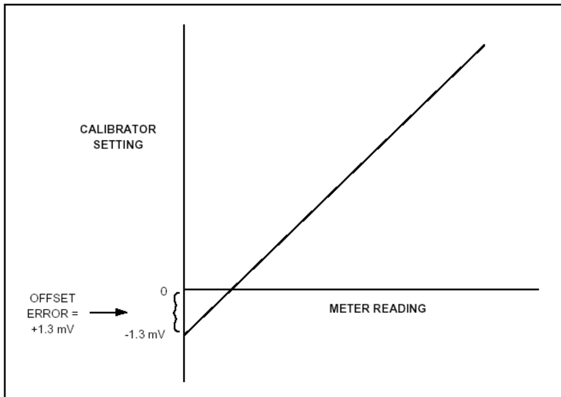
图4-7. 偏置误差
