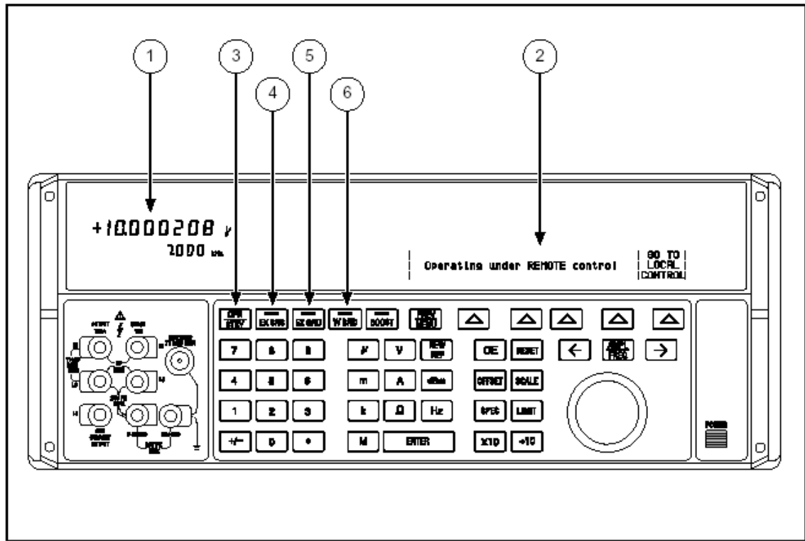
3-1. 前面板功能
