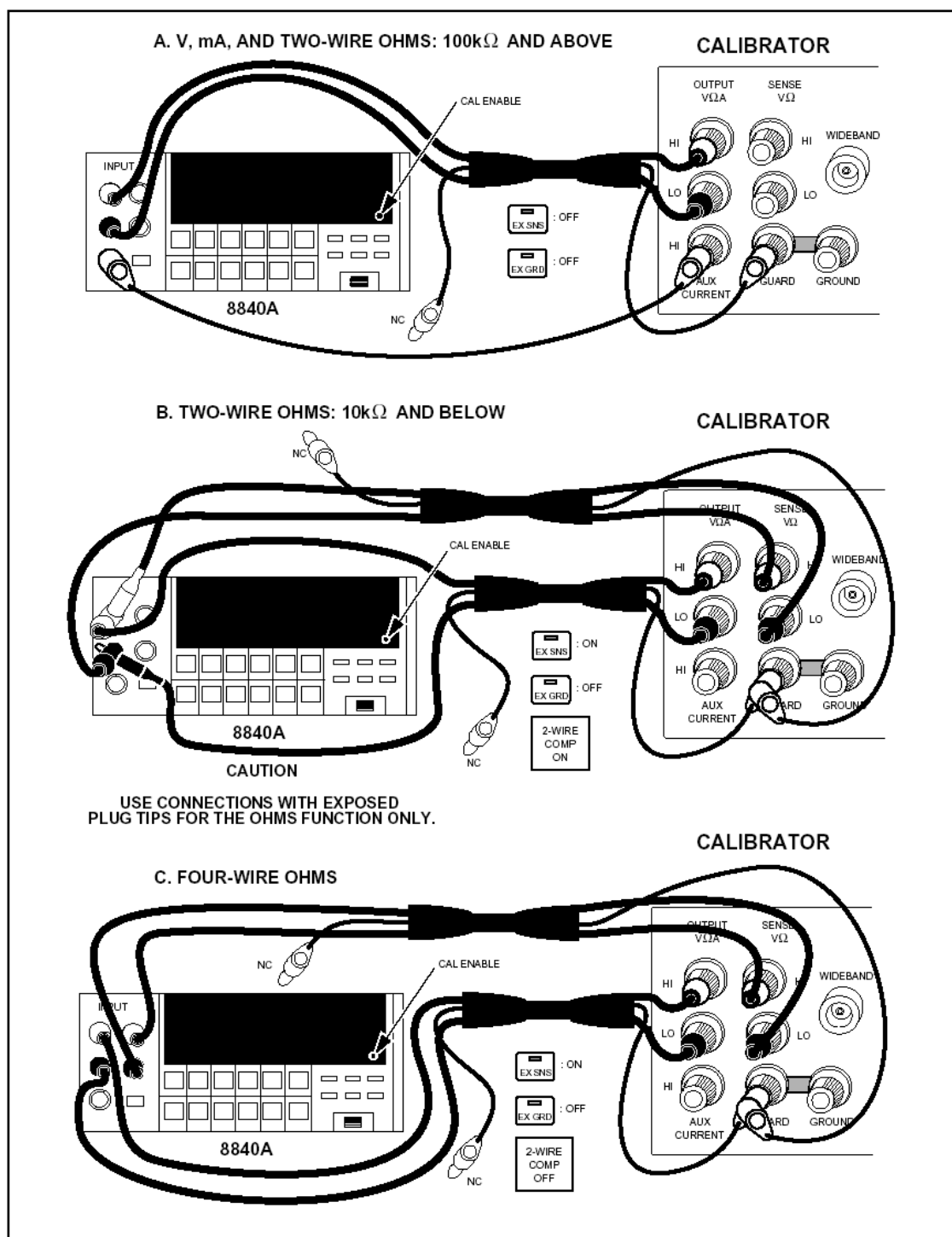
图4-13. 8840A多用表的校准连接
