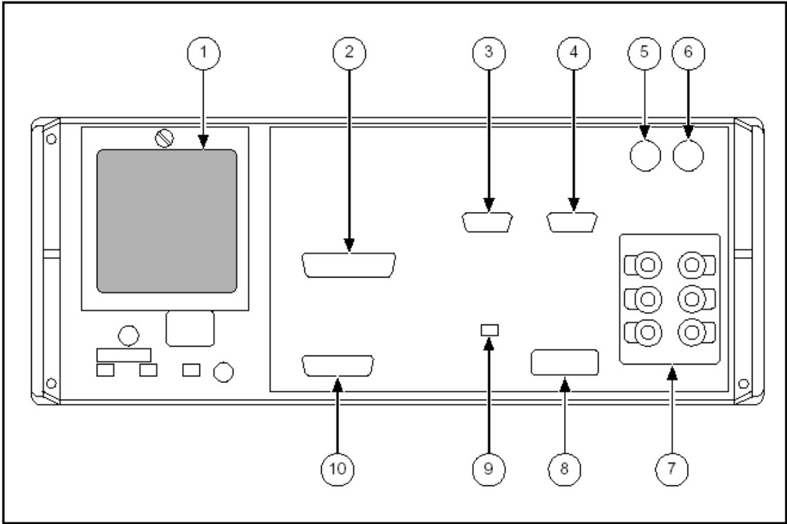
图3-2. 后面板功能
