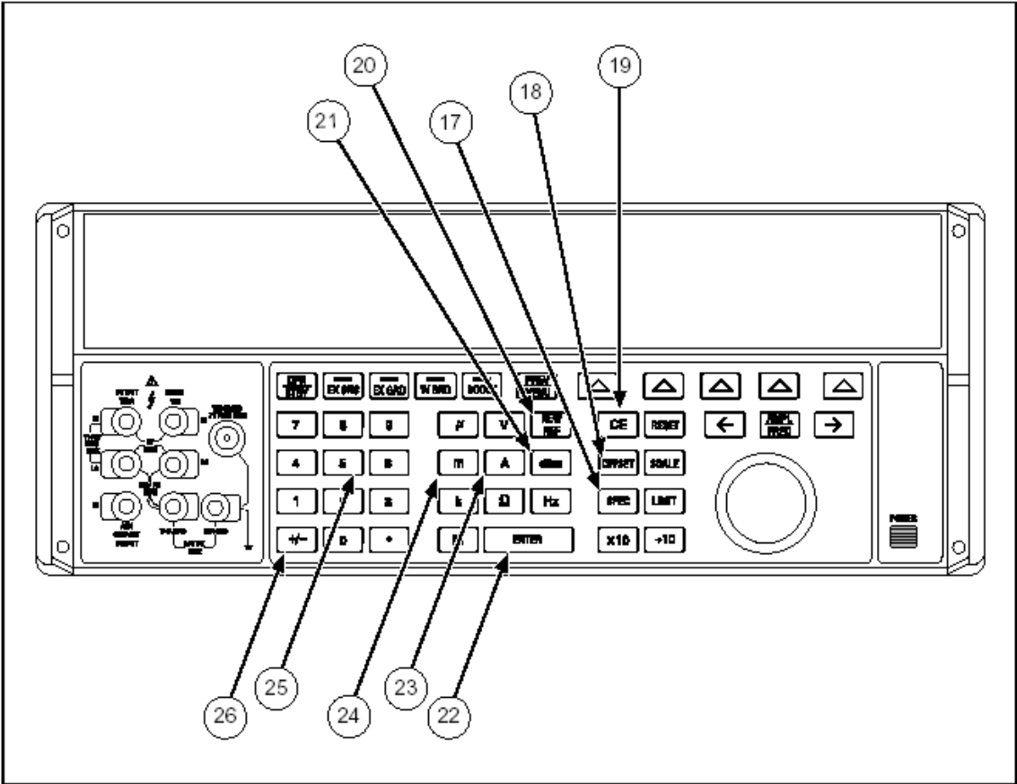
图3-1. 前面板功能(续)
