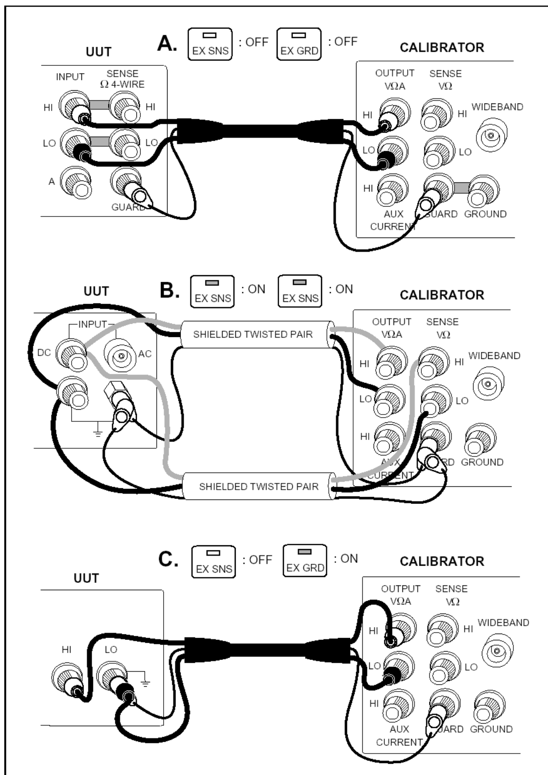
图4-1. UUT连接方法: 直流电压, 交流电压 \leq 10 kHz
