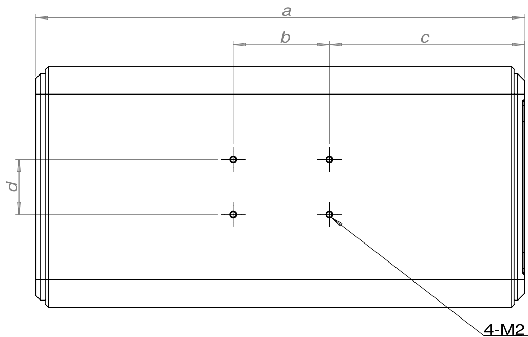
俯视图
