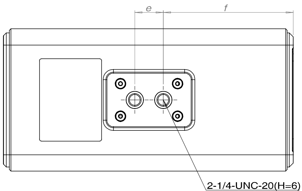
仰视图
