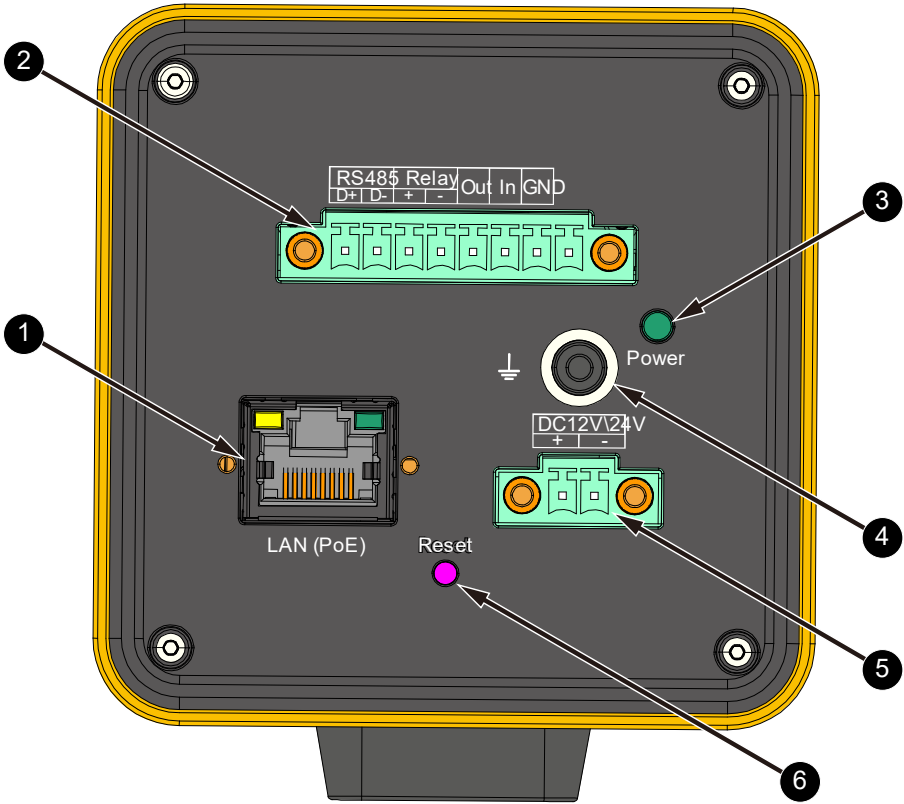
图 5. 产品接口
