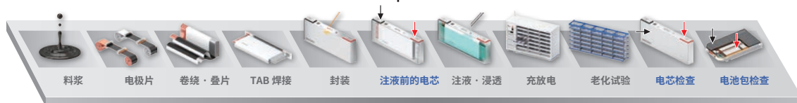
锂电池生产线的工序示意图
