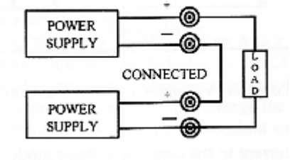
图 5-2 两个电源供应器串联工作
