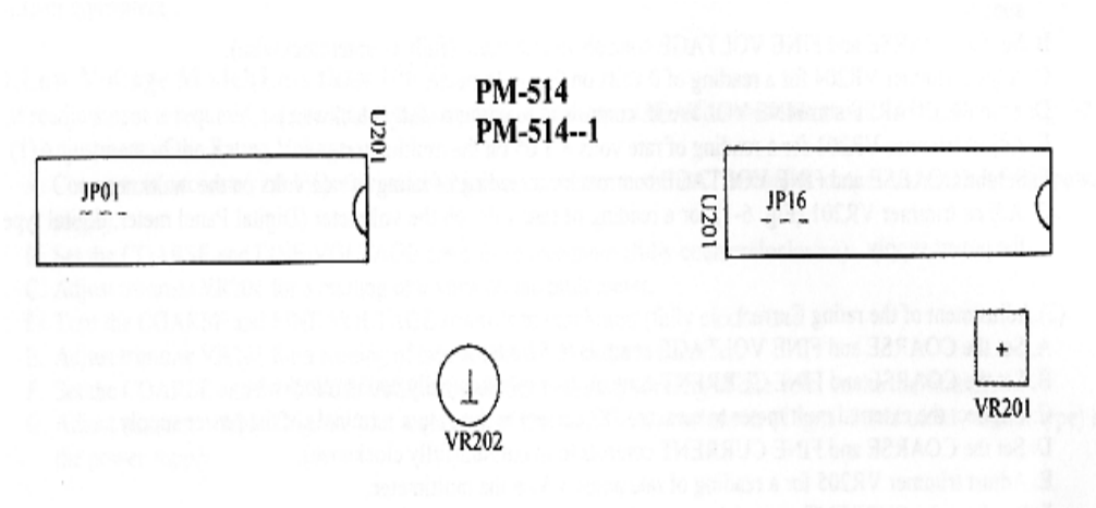
图 6-1 调节位置
