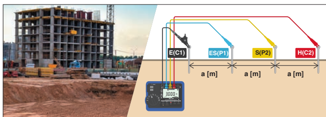
4电极法 适用于测量接地设计所需的大地电阻率
