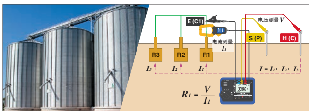
MEC功能 适用于在不切断接地极的情况下测量接地电阻
