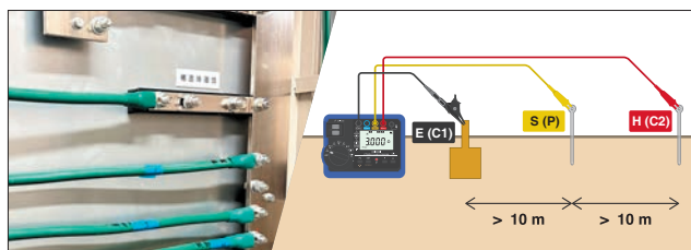
3电极法 适用于精确测量接地电阻
