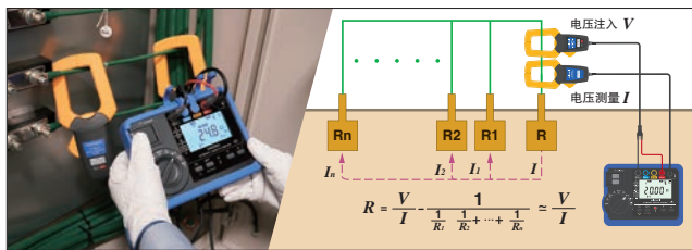
钳式测试法(双钳式) 适用于测量多重接地的接地电阻
