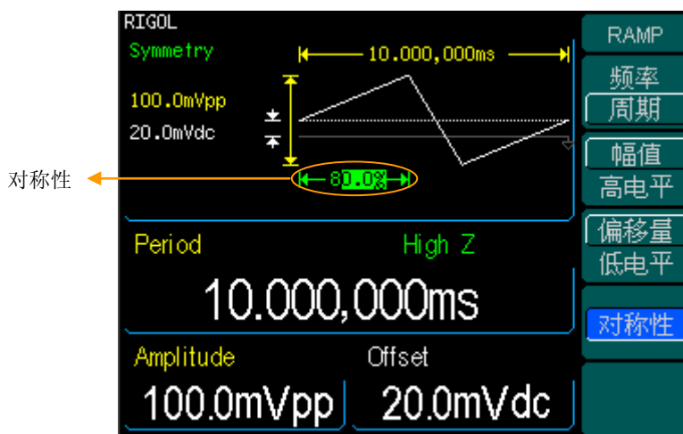
图 2-9 锯齿波形及参数值显示窗口
