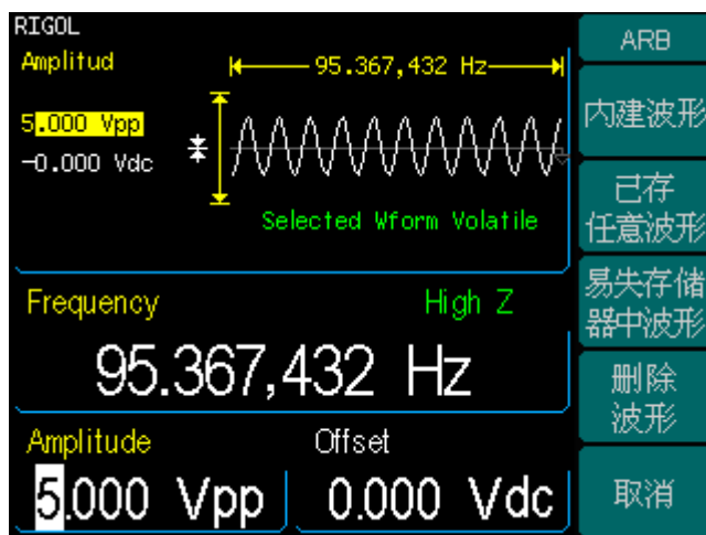
图 2- 61 读取波形
