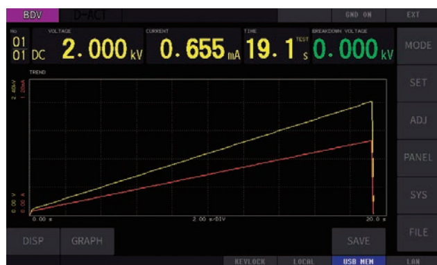
连续升压测试示例
