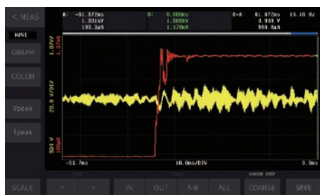
仅放大波形显示
