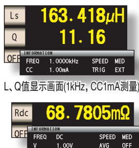
Rdc显示画面(DC测量)
