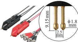
针型探头 L2003 线长1.5 m
