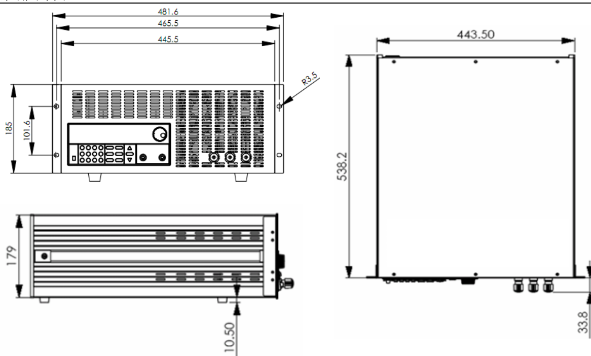
详细尺寸图
