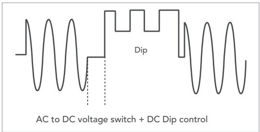
AC/DC server PSU测试需求 (电压波形)
