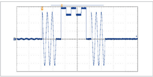
61509实际输出电压波形
