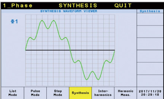
Waveform Viewer呈现谐波合成功能
