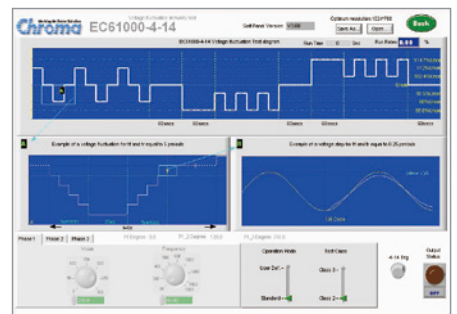
電壓波動抗擾度測試
