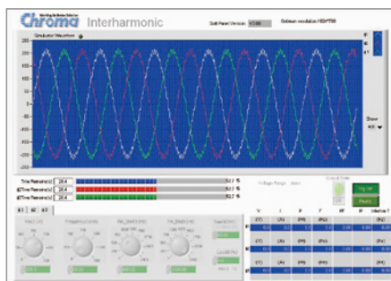
間諧波測試
