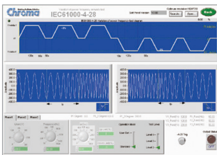
頻率變化抗擾度測試
