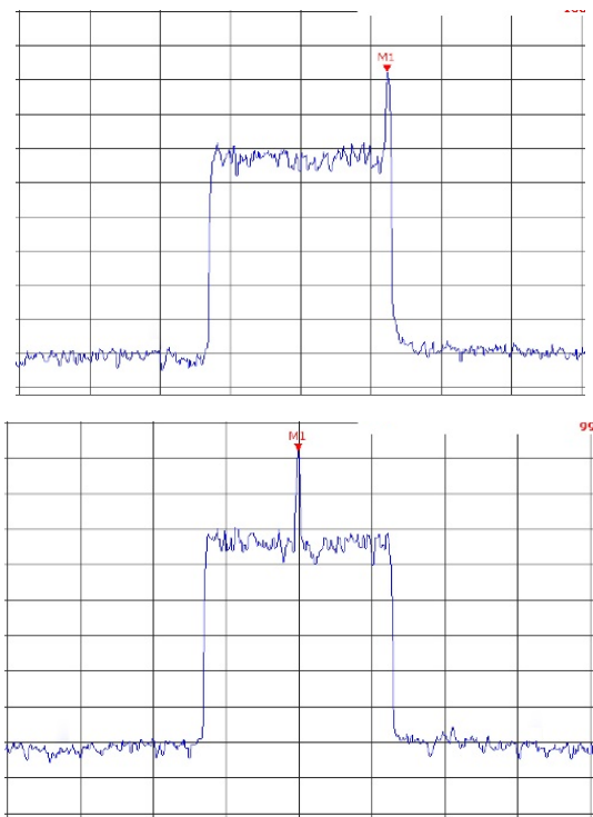
(a) LoS AoA = 0 ° (b) LoS AoA = 90 °
