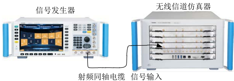
图 5.5 实时衰落引擎测试图
