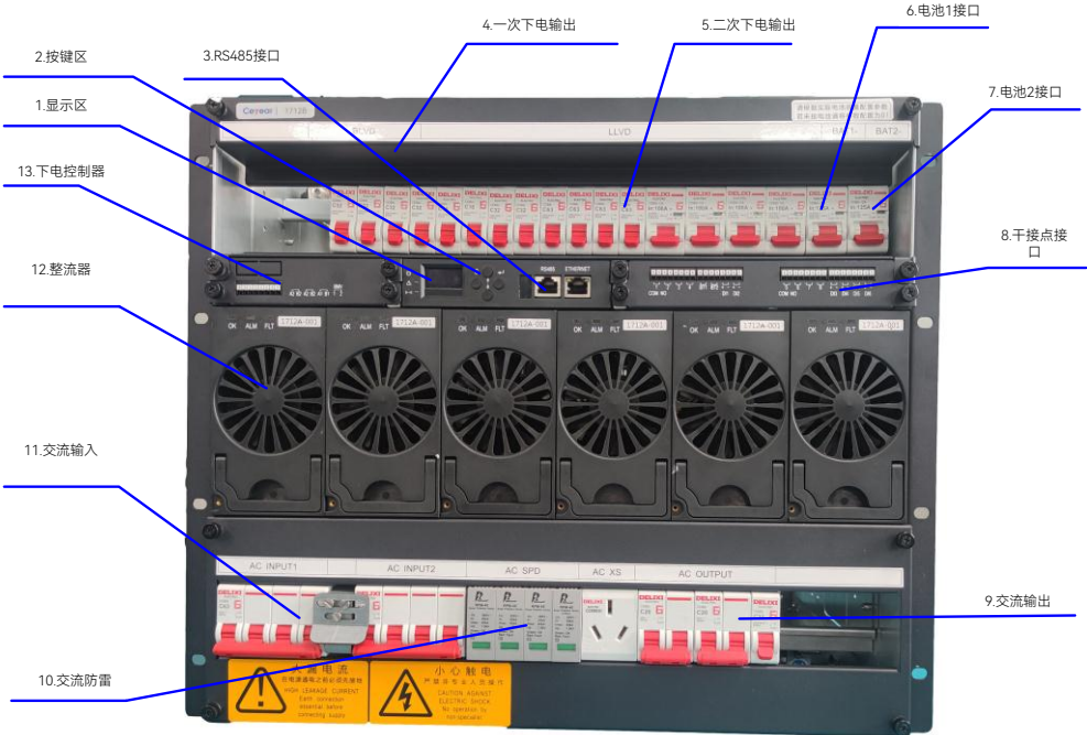
图 4.1 1712A/B 前面板
