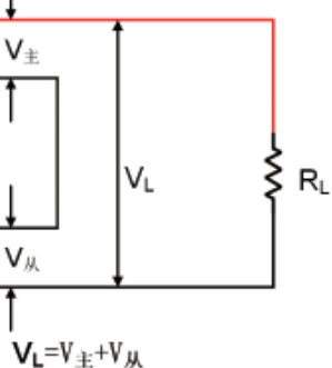
串联模式电压相加
