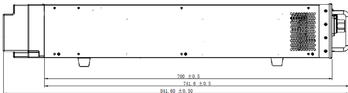
IT7842E-350-210 机型
