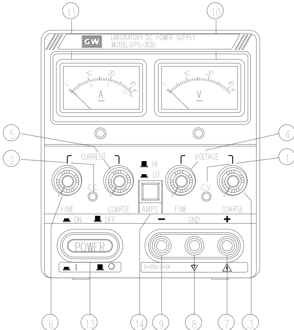
● 圖 4-2 前面板(類比式)
