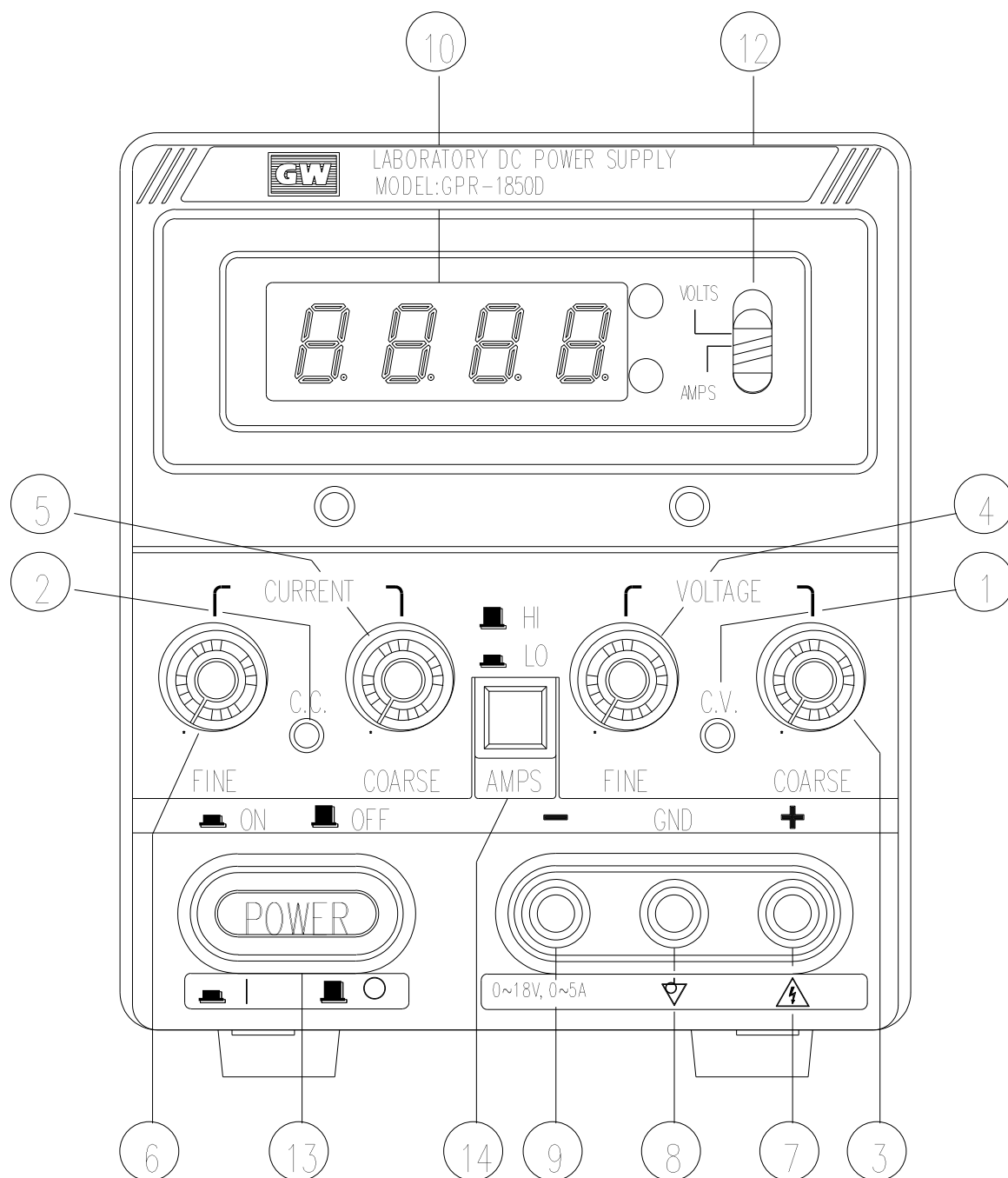
● 圖 4-1 前面板(數字式)
