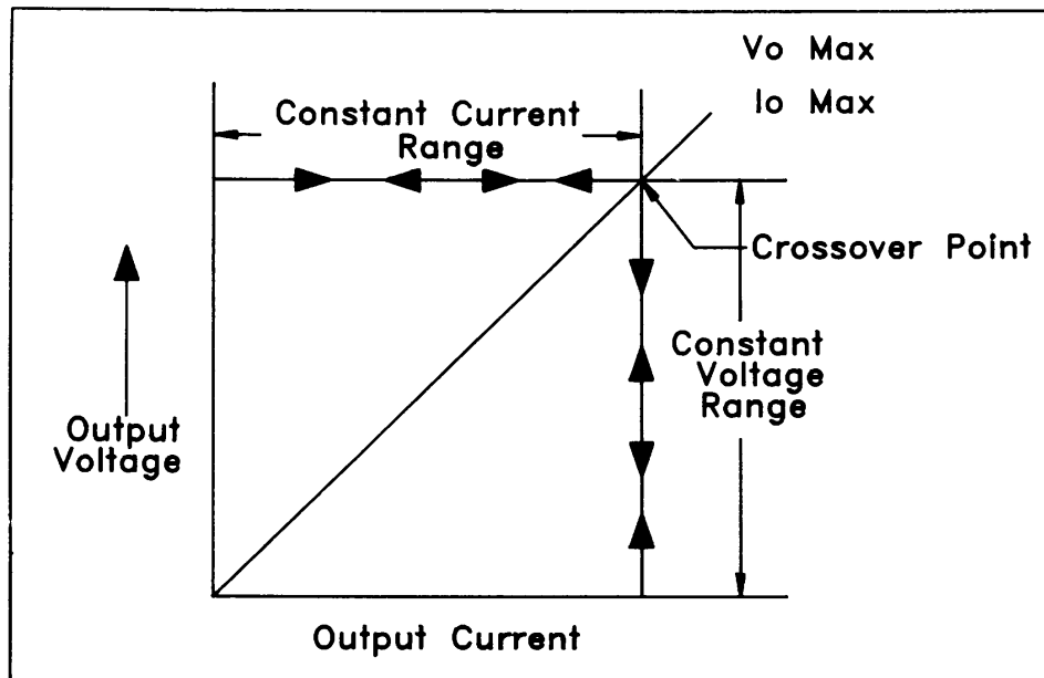
● 圖 5-1 定電壓/定電流特性
