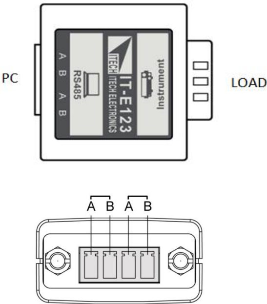
RS485接口引脚
